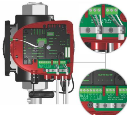
Kuva 5. Pumppu sisältä (Grundfos)
