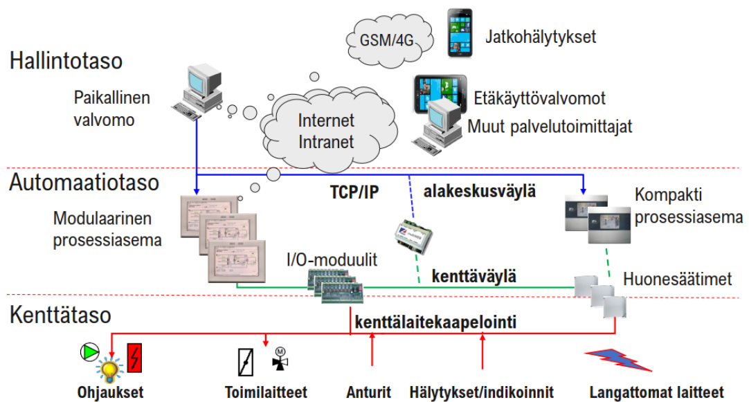
Kuva 1. Automaatiojärjestelmän rakenne (ST-Käsikirja 17, s. 60)
