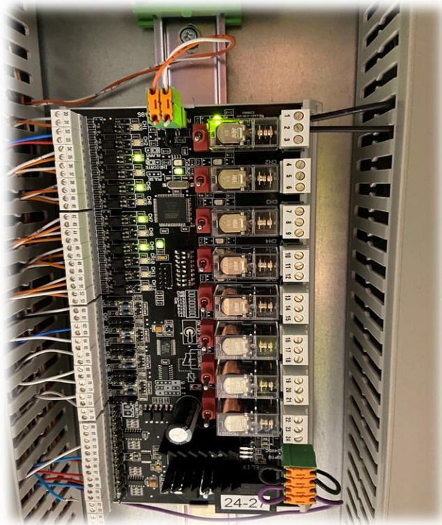
Kuva 16. DIN-kiskoasenteinen yhdistelmämoduuli COMBI-36.
