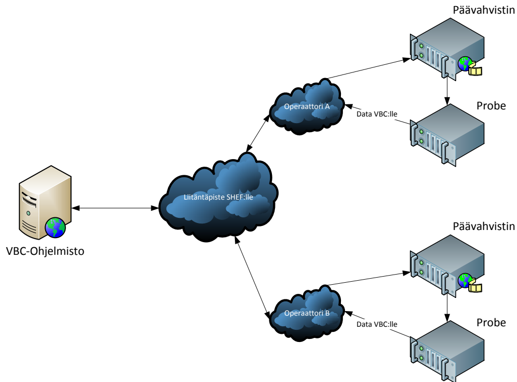
KUVIO 5: Bridgetech järjestelmän topologia.
