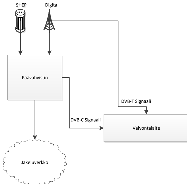
KUVIO 6: Laitteen asentaminen päävahvistimeen.
