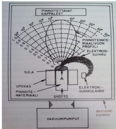
Kuvio 12. Höyrystysprosessin periaatekuva. /26, 129/
