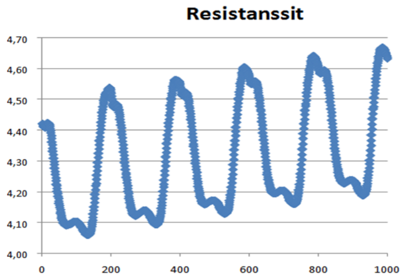
KUVA 13. Johtimen resistanssin muutokset kompressiotaivutuksen aikana
