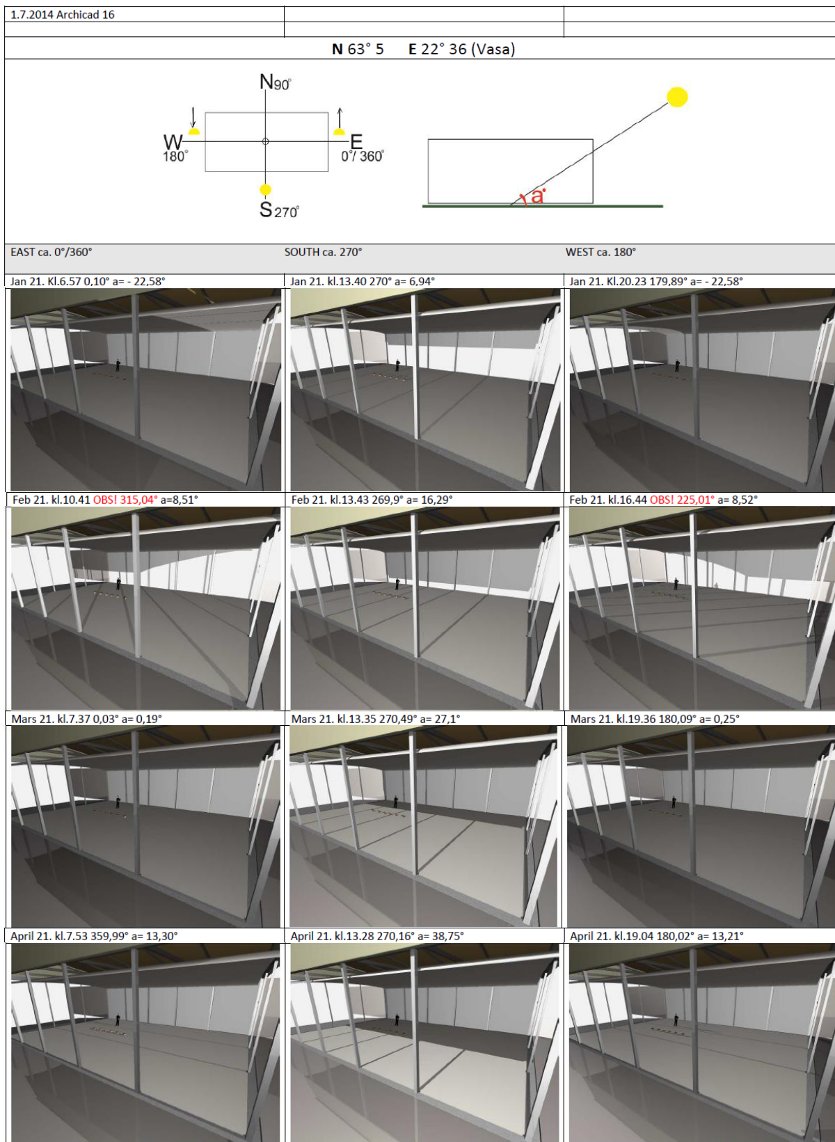
Bilaga 2. Simulerade 3D-skuggbilder för konceptväxthuset utan sockel för den 21 i varje månad under ett år när solen står som högst i öst, syd och väst.
