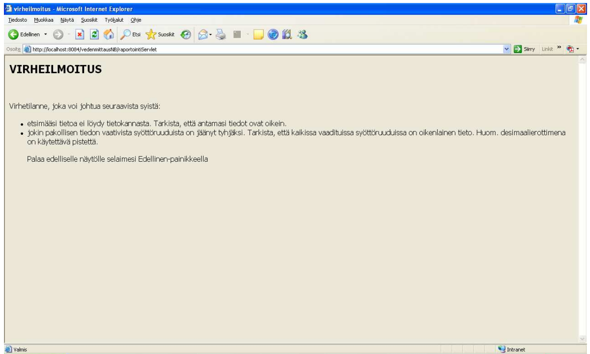
Kuvio 17. Virheilmoitus-käyttöliittymä
