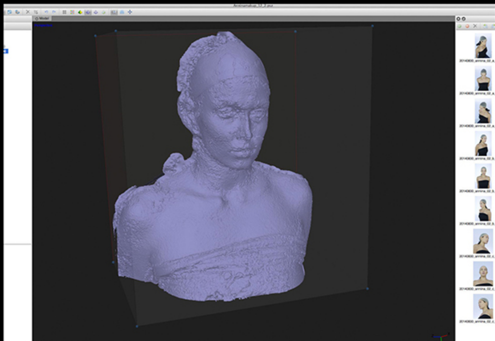
Polygonimesh kuvista
