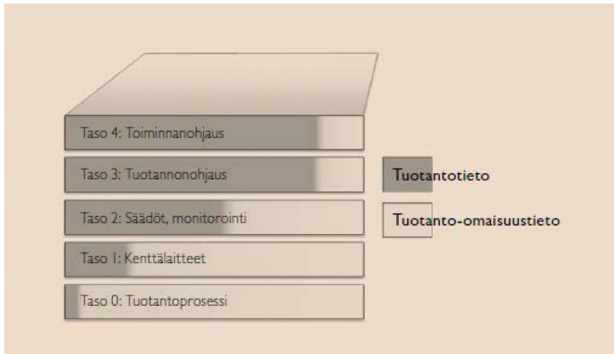
Kuva 21. IEC 62264 standardin toiminnallisen hierarkian tasot (Marttinen 2012, 20.)
